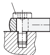
DIN 732.1 柱头带肩螺栓 用作轴承销
